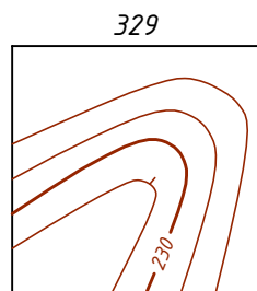
Хребет
