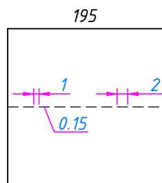
Тропа
