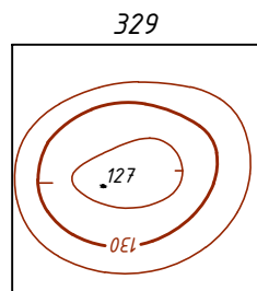
Котловина
