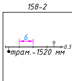
Трамвайные линии
