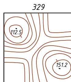
Седловина
