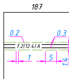
Шоссе усовершенствованное
