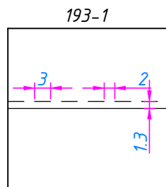
Проселочная дорога
