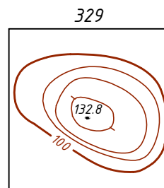
Гора
