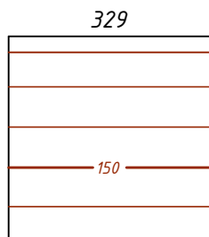
Ровный склон
