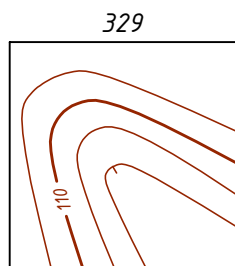
Лощина
