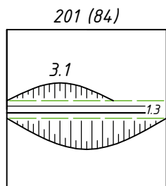
Дороги в выемках
