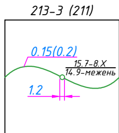
Отметка уреза воды
